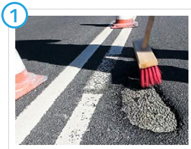
1 Staub und losen Schmutz im Einsatzbereich gründlich entfernen.
