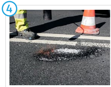
4 Erhitzen Sie das Material auf ca. 200°C mit dem Gasbrenner.
